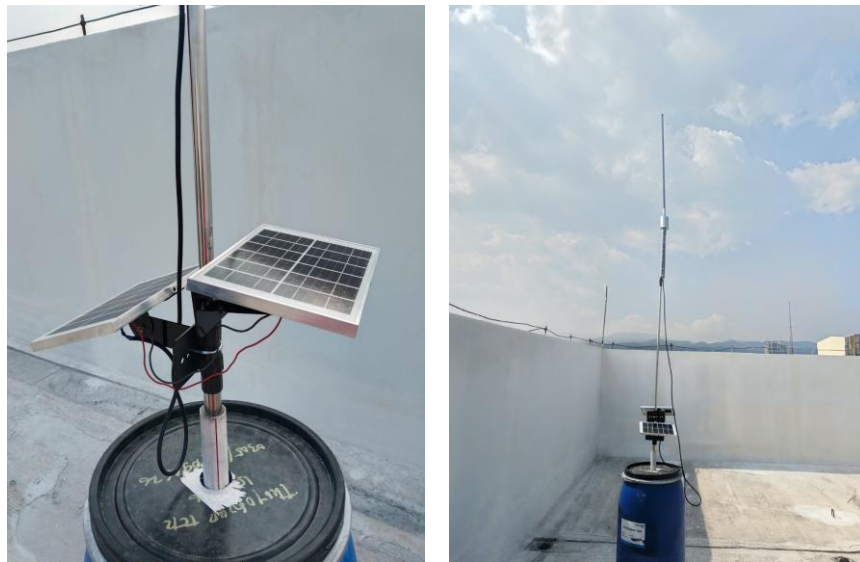
Gambar 3.1 Konfigurasi Cluster Head: bracket 2 panel surya diklem ke tiang (kiri), unit CH & antena di bagian atas tiang (kanan). Foto uji LGU & ITB; drum hanya kedudukan sementara — di RU IV tiang ditanam & dicor.
